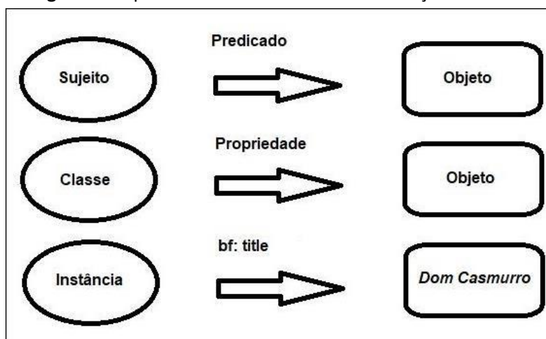
Figura 2: Esquema de estrutura de uma declaração Bibframe
